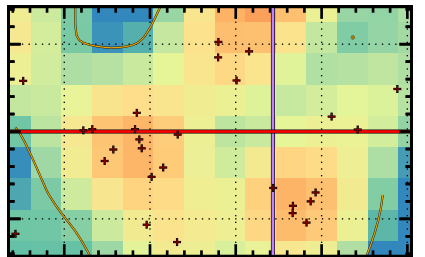
Pisces-Cetus
